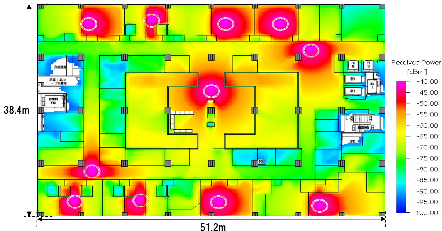
電磁界シミュレーションによる導入前無線LAN到達範囲調査
